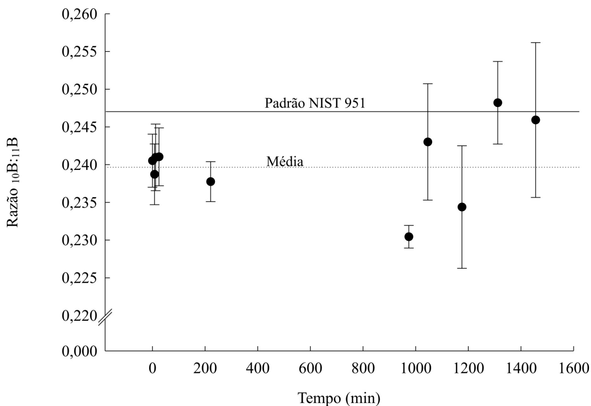
Figura 1S. Razão isotópica de B, considerando o tempo de duração das séries analíticas
